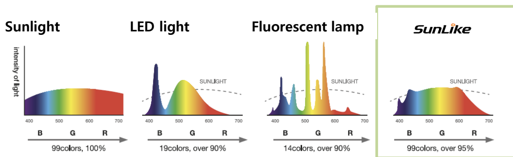
[스펙트럼 비교]
